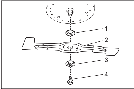
► 1. Brida interior 2. Cuchilla de la cortadora de césped 3. Brida exterior 4. Perno
